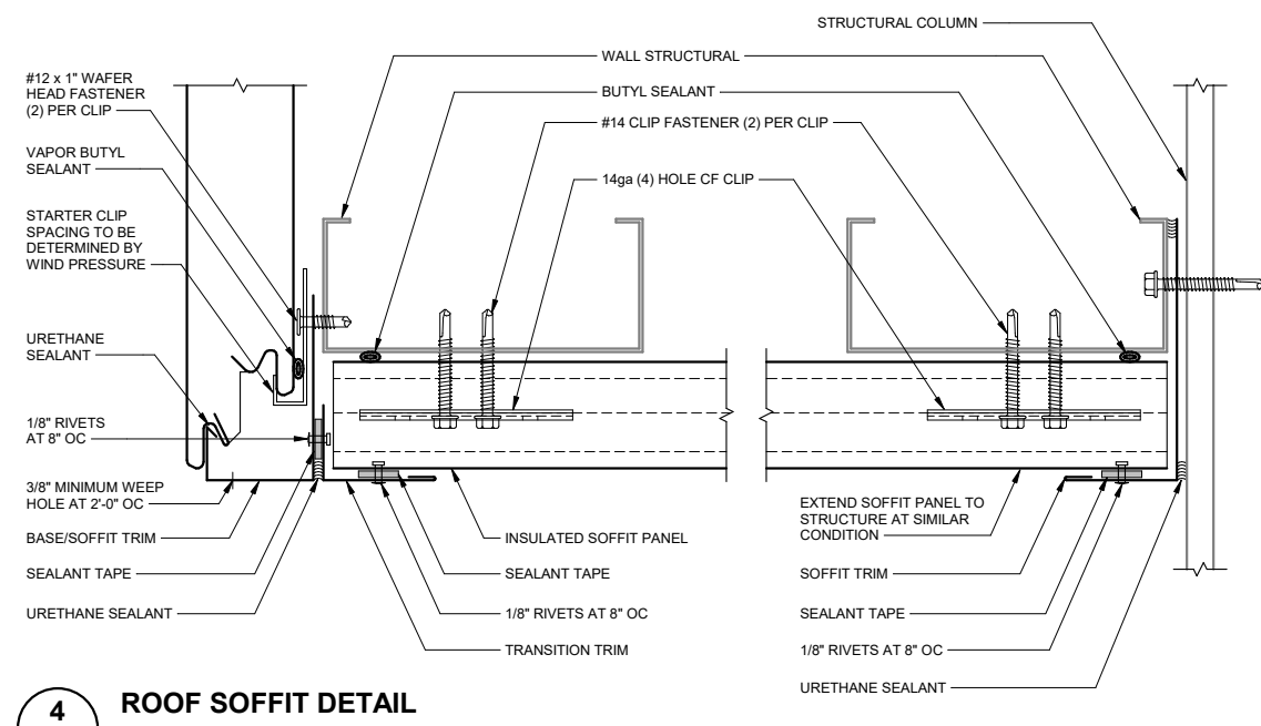
4 ROOF SOFFIT DETAIL A-302 SCALE: 6" = 1'-0"
